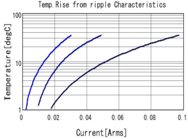
GRM188R72E102KW07 Temp. rise ■ 30kHz ■ 100kHz ■ 300kHz
