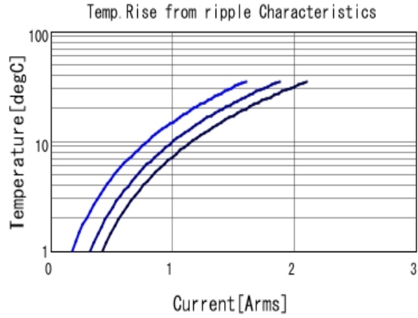
GRM188R71H154KAC4 Temp. rise ■ 400kHz ■ 800kHz ■ 1MHz
