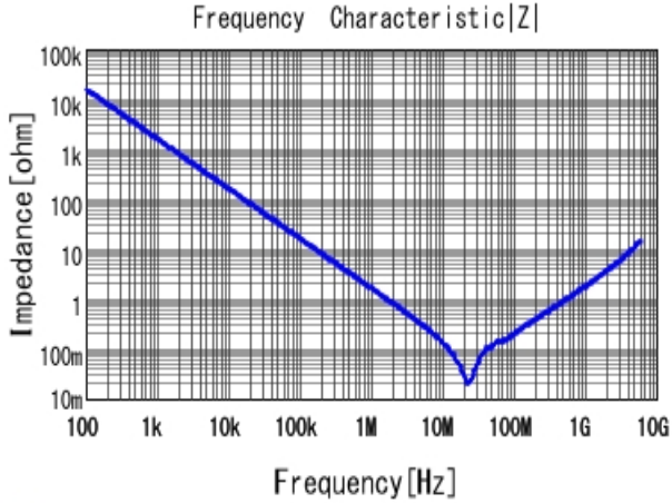
■ GRM188R71H104KA93 |Z| DCOV, 25degC
