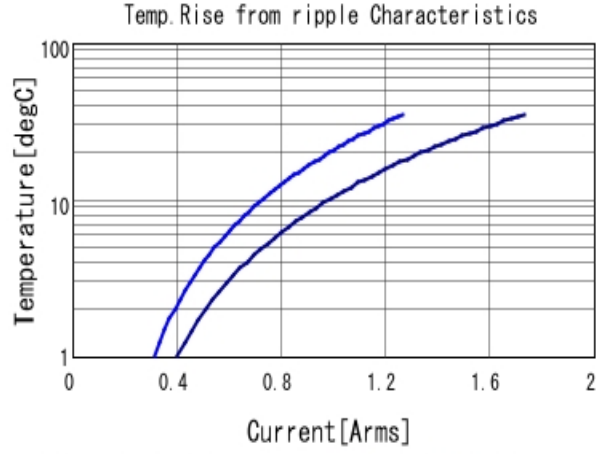
GRM188R71H104KA93 Temp. rise ■ 500kHz ■ 1MHz
