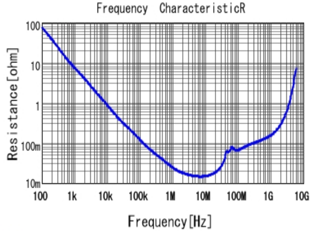
■ GRM188R71H104KA93 R DCOV, 25degC
