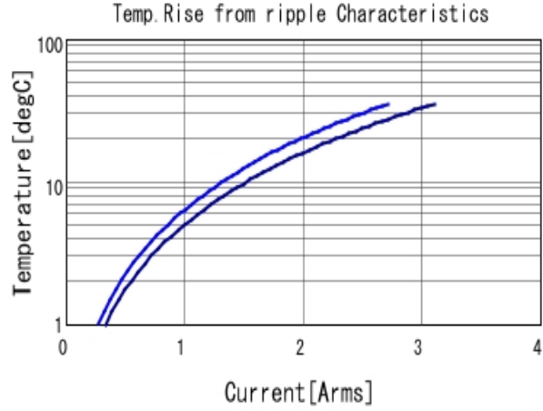
GRM188R71E105KA12 Temp. rise ■ 500kHz ■ 1MHz
