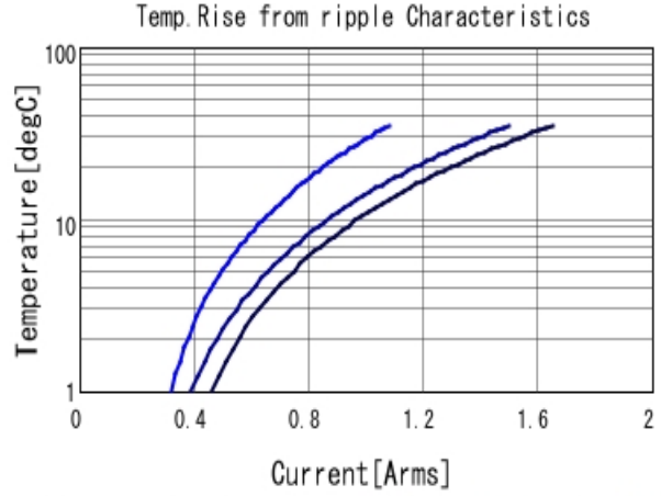
GRM188R71E104KA01 Temp. rise ■ 400kHz ■ 800kHz ■ 1MHz
