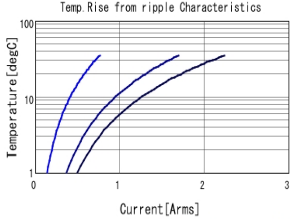
GRM188R71A684KA61 Temp. rise ■ 100kHz ■ 500kHz ■ 1MHz
