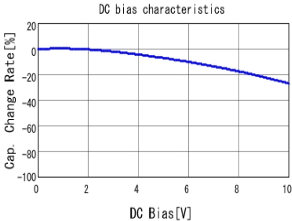
■ GRM188R71A684KA61 C-DC bias capchange, 25.0degC, AC1.
