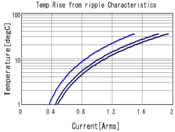
GRM188R71A334KA61 Temp. rise ■ 300kHz ■ 600kHz ■ 1MHz
