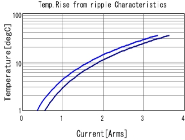
GRM188R71A225KE15 Temp. rise ■ 500kHz ■ 1MHz
