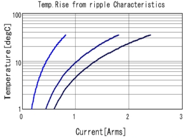
GRM188R71A224KA01 Temp. rise ■ 100kHz ■ 500kHz ■ 1MHz
