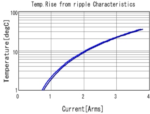
GRM188R61H225KE11 Temp. rise ■ 500kHz ■ 1MHz
