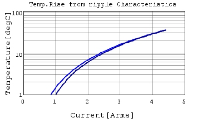
GRM188R61E475KE11 Temp.rise — 500kHz
