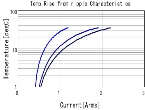
GRM188R61E474KA12 Temp. rise ■ 200kHz ■ 500kHz ■ 1MHz
