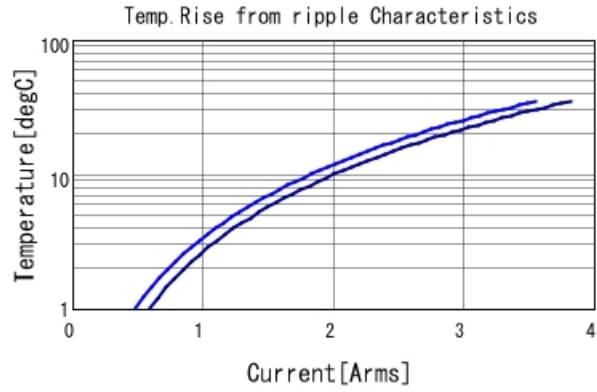
GRM188R61E225MA12 Temp. rise ■ 500kHz ■ 1MHz
