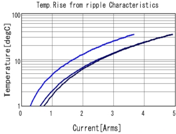
GRM188R61E106MA73 Temp. rise ■ 80kHz ■ 400kHz ■ 800kHz
