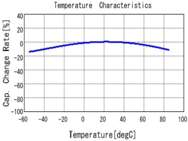
■ GRM188R61E106MA73 C-Temp. capchange, DCO. 0V, ACO. 2V rm
