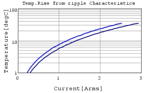
GRM188R61E105KA12 Temp.rise — 500kHz —
