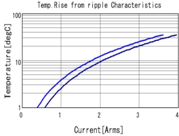
GRM188R61C225KE15 Temp. rise ■ 500kHz ■ 1MHz
