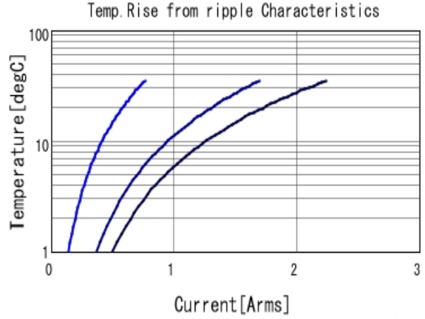
■ GRM188R61A684KA61 Temp. rise ■ 100kHz ■ 500kHz ■ 1MHz
