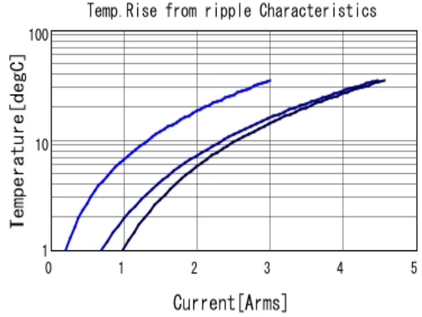
GRM188R61A475KE15 Temp. rise ■ 100kHz ■ 500kHz ■ 1MHz
