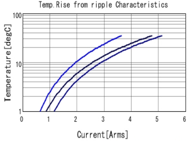
GRM188R61A475KAAJ Temp. rise ■ 100kHz ■ 500kHz ■ 1MHz
