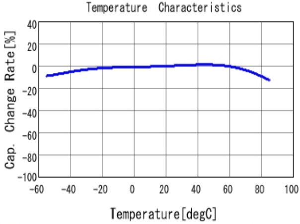
■ GRM188R61A226ME15 C-Temp. capchange, DCO. 0V, ACO. 2V rm
