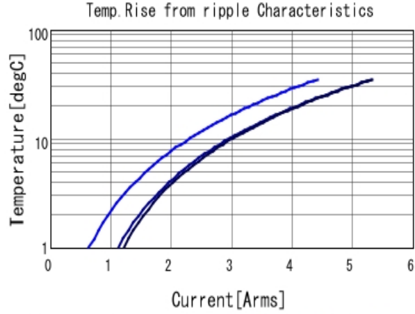
GRM188R61A226ME15 Temp. rise ■ 80kHz ■ 400kHz ■ 800kHz
