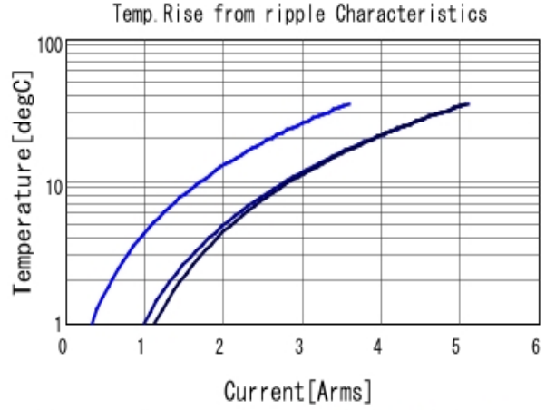
GRM188R60J106ME47 Temp. rise ■ 80kHz ■ 400kHz ■ 800kHz
