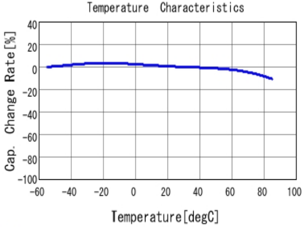
■ GRM188R60J106ME47 C-Temp. capchange, DCO. 0V, ACO. 5V rm
