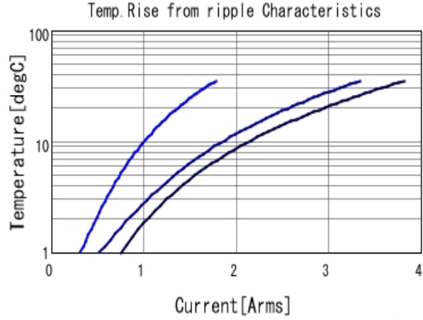
GRM188R60J105KA01 Temp. rise ■ 100kHz ■ 500kHz ■ 1MHz
