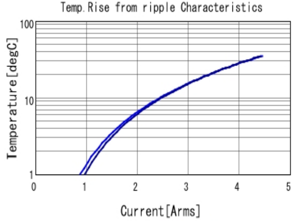
GRM188D71A475KE11 Temp. rise ■ 500kHz ■ 1MHz
