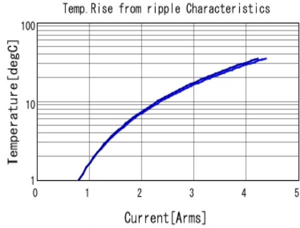
GRM188C81E475KE11 Temp. rise ■ 500kHz ■ 1MHz
