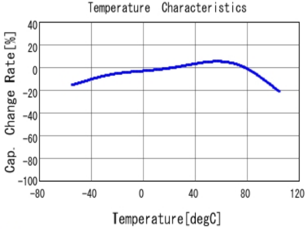
■ GRM188C80J226ME15 C-Temp. capchange, DCO. 0V, ACO. 1Vrm
