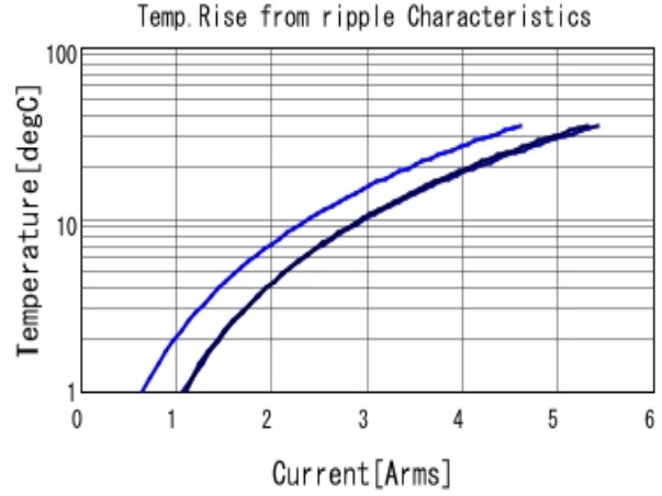
GRM188C80J226ME15 Temp. rise ■ 80kHz ■ 400kHz ■ 800kHz
