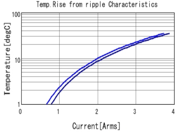
GRM188C71E225KE11 Temp. rise ■ 500kHz ■ 1MHz
