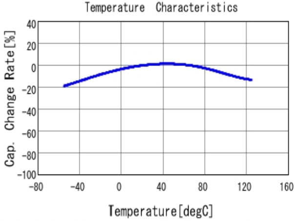
■ GRM188C71E225KE11 C-Temp. capchange, DCO. 0V, ACO. 2V rm
