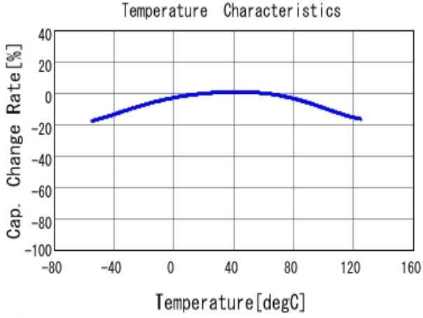
■ GRM188C71A475KE11 C-Temp. capchange, DCO. 0V, ACO. 2V rm
