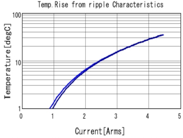
GRM188C71A475KE11 Temp. rise ■ 500kHz ■ 1MHz
