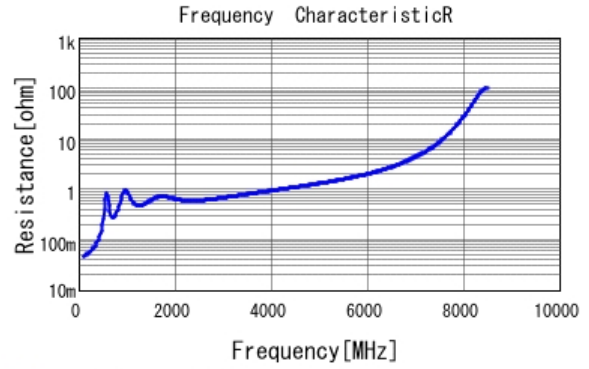
■ GRM1885C1H561JA01 R DCOV, 25degC
