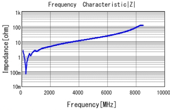
■ GRM1885C1H561JA01 |Z| DCOV, 25degC
