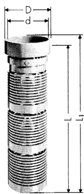
DN 65–100
