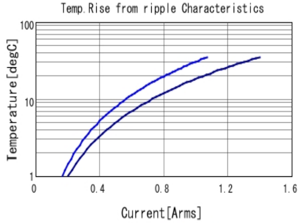
GRM155R71H104KE14 Temp. rise ■ 500kHz ■ 1MHz
