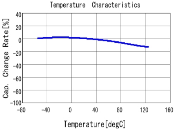
■ GRM155R71H104KE14 C-Temp. capchange, DCO. 0V, AC1.0V rm
