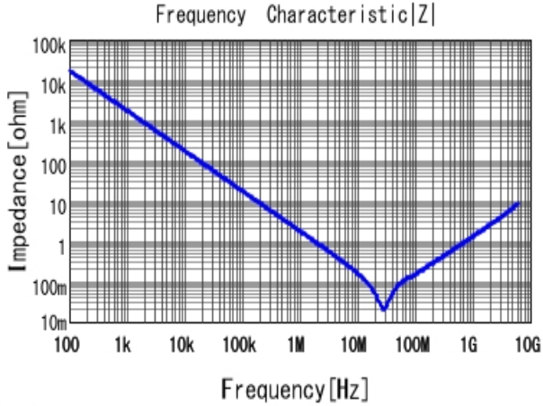
■ GRM155R71H104KE14 |Z| DCOV, 25degC
