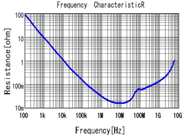
■ GRM155R71H104KE14 R DCOV, 25degC
