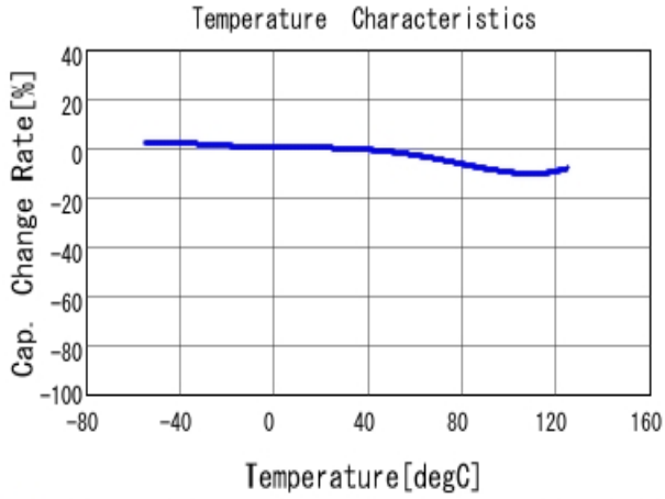
■ GRM155R71E222KA01 C-Temp. capchange, DCO. 0V, AC1.0Vrm
