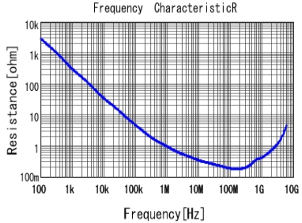
■ GRM155R71E222KA01 R DCOV, 25degC
