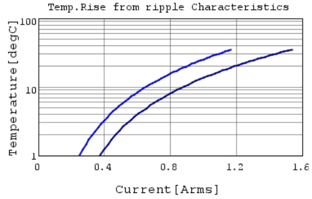
GRM155R71E104ME14 Temp.rise — 500kHz —
