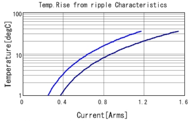
GRM155R71E104KE14 Temp. rise — 500kHz — 1MHz
