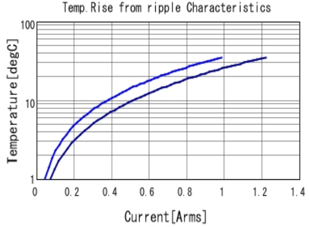
GRM155R71C154KA12 Temp. rise ■ 500kHz ■ 1MHz
