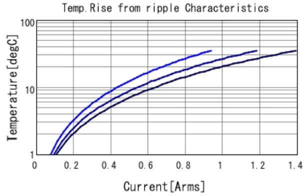
GRM155R71A224KE01 Temp. rise — 300kHz — 600
