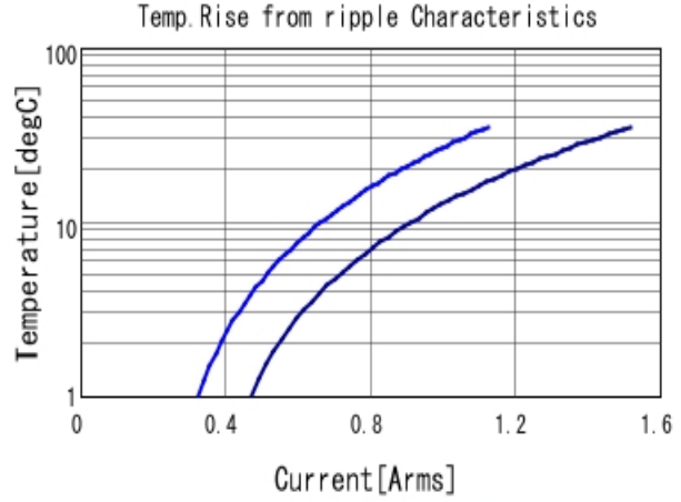
GRM155R71A104KA01 Temp. rise ■ 500kHz ■ 1MHz
