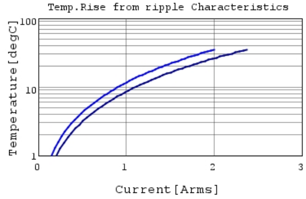
GRM155R70J105KA12 Temp.rise — 500kHz —
