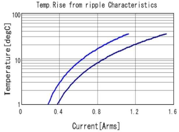
GRM155R70J104KA01 Temp. rise ■ 500kHz ■ 1MHz
