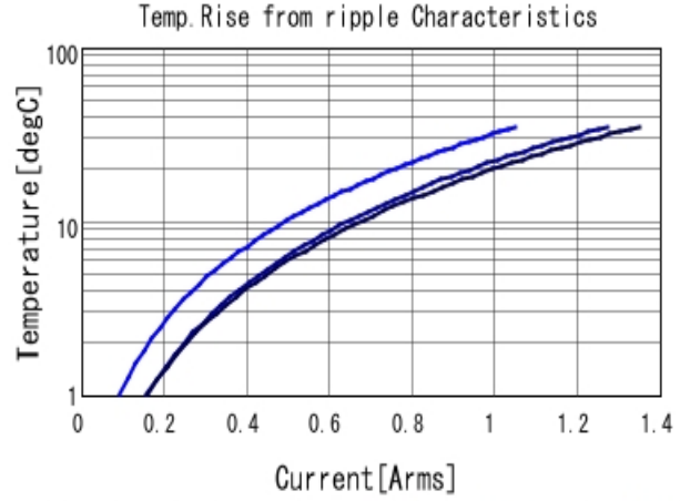
GRM155R62A104KE14 Temp. rise ■ 400kHz ■ 800kHz ■ 1MHz
