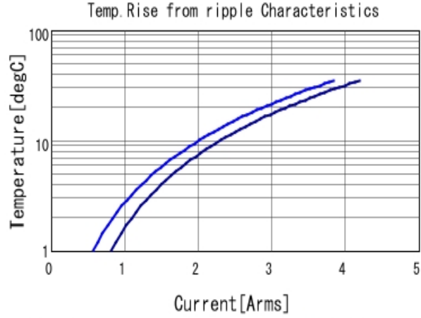
GRM155R61E225ME15 Temp. rise ■ 500kHz ■ 1MHz
