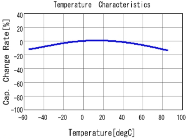
■ GRM155R61E225ME15 C-Temp. capchange, DCO. 0V, ACO. 2V rm
