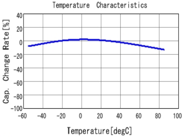
■ GRM155R61E225KE11 C-Temp. capchange, DCO. 0V, ACO. 2V rm
