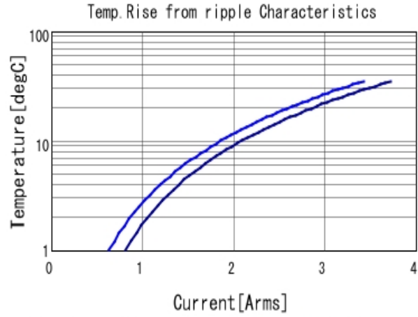
GRM155R61E225KE11 Temp. rise ■ 500kHz ■ 1MHz
