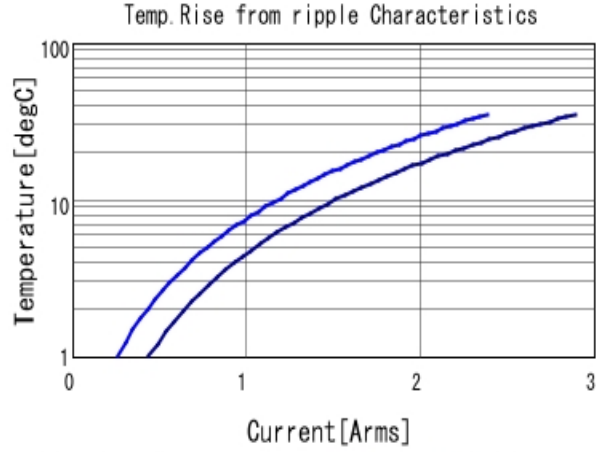
GRM155R61E105MA12 Temp. rise ■ 500kHz ■ 1MHz
