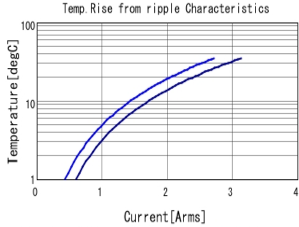
GRM155R61E105KE11 Temp. rise ■ 500kHz ■ 1MHz
