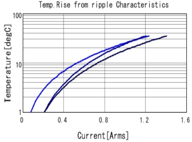
GRM155R61E104MA87 Temp. rise ■ 400kHz ■ 800kHz ■ 1MHz
