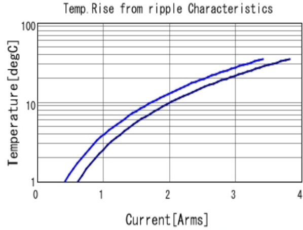
GRM155R61C225KE44 Temp. rise ■ 500kHz ■ 1MHz
