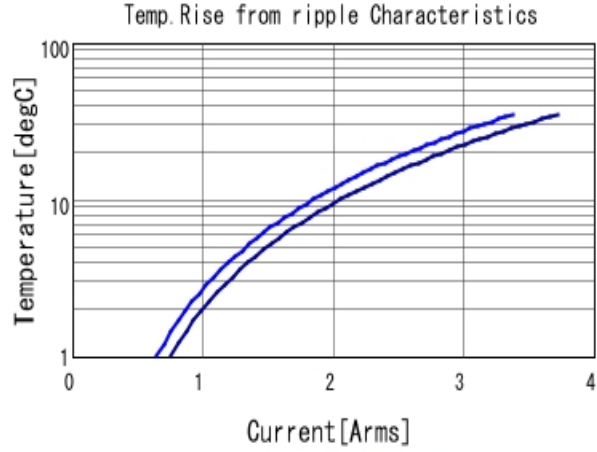
GRM155R61C225KE11 Temp. rise ■ 500kHz ■ 1MHz
