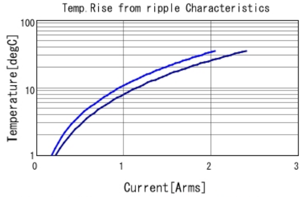
GRM155R61C105KA12 Temp. rise ■ 500kHz ■ 1MHz
