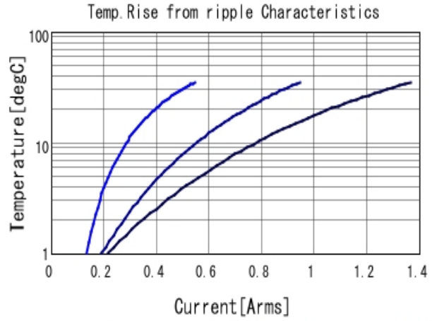
GRM155R61C104KA88 Temp. rise ■ 100kHz ■ 500kHz ■ 1MHz
