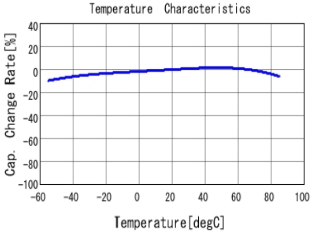
■ GRM155R61A475MEAA C-Temp. capchange, DCO. 0V, ACO. 1Vrm
