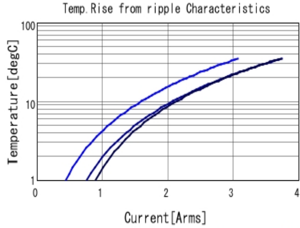
GRM155R61A475MEAA Temp. rise ■ 100kHz ■ 500kHz ■ 1MHz
