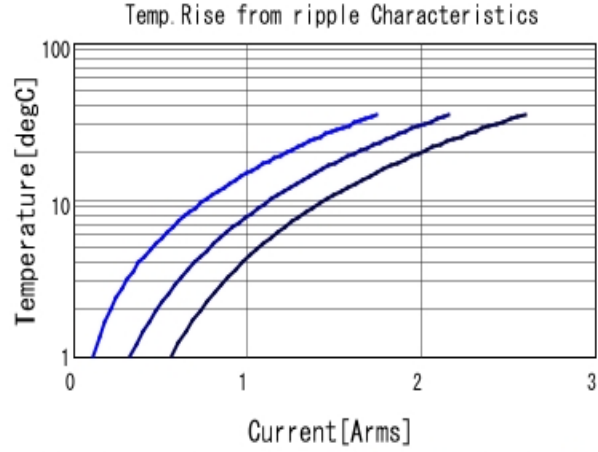
GRM155R61A474KE15 Temp. rise ■ 100kHz ■ 500kHz ■ 1MHz
