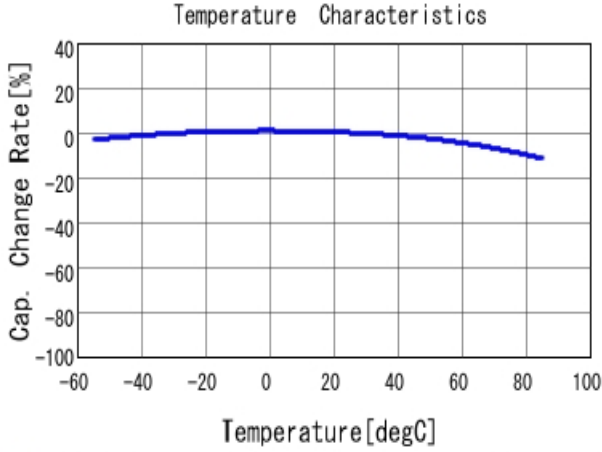
■ GRM155R61A474KE15 C-Temp. capchange, DCO. 0V, ACO. 5V rm
